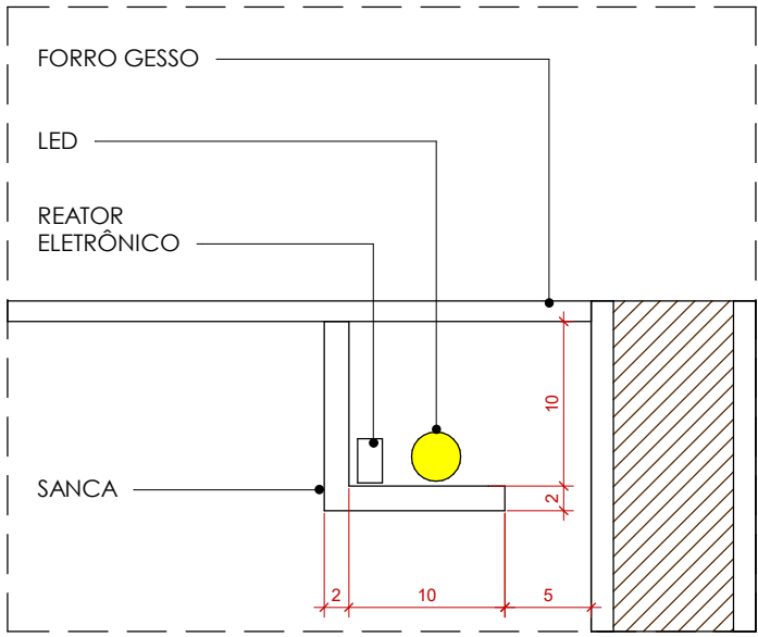
Det. Sanca - TIPO A 1 : 5
