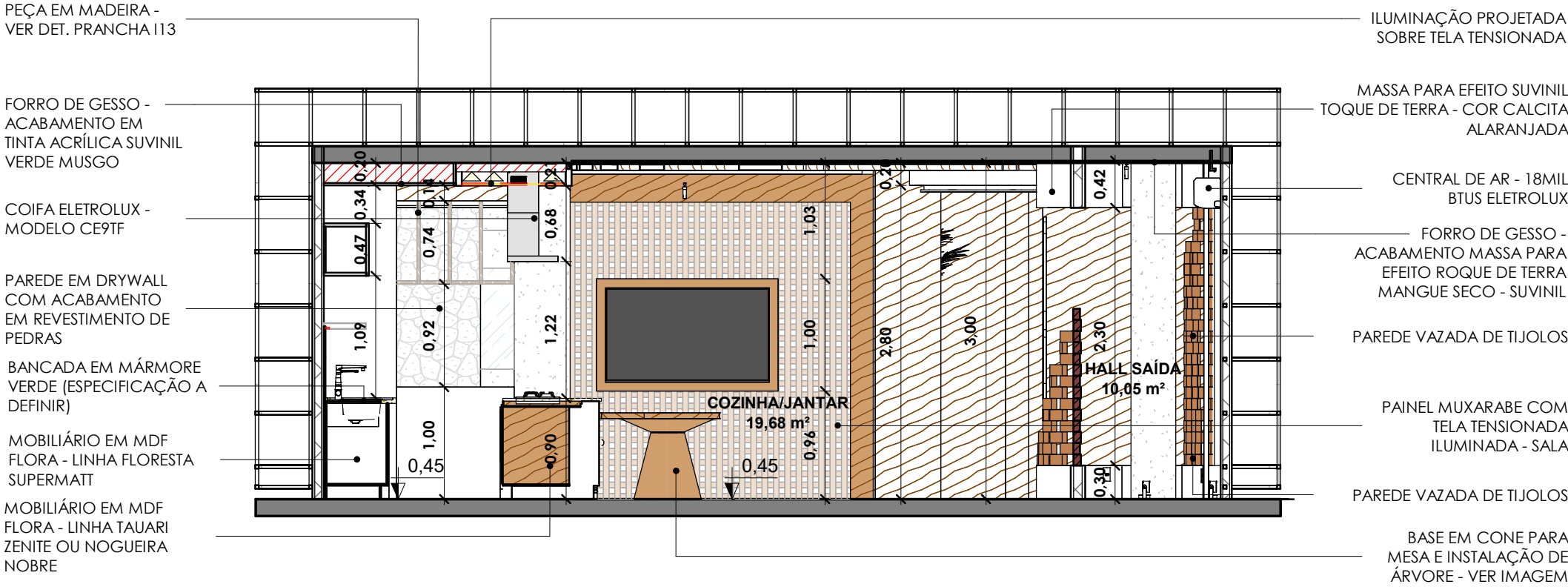
CORTE C 1 : 50
