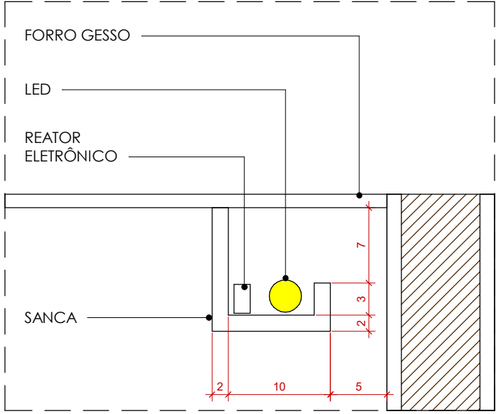
Det. Sanca - TIPO B 1 : 5
