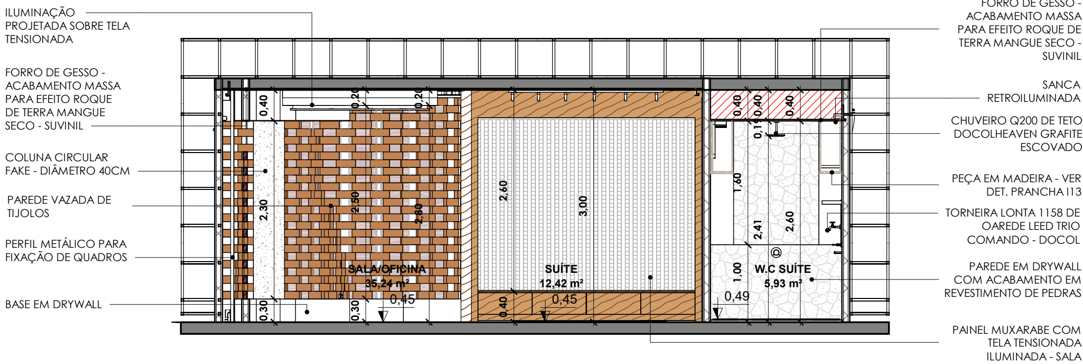
CORTE D 1 : 50
